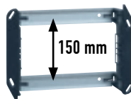
Châssis à rattrapage d'aplomb. Corrige le niveau d'une boîte d'encastrement. Espace entre les rails à l'entraxe de 150 mm
